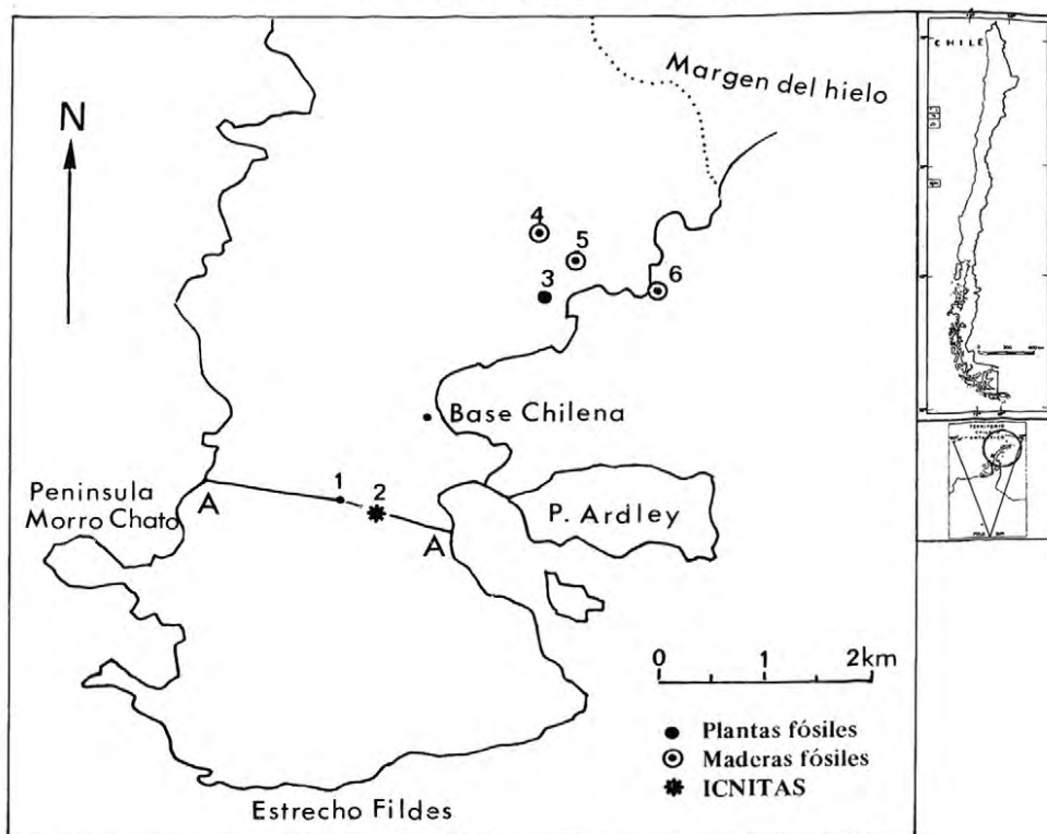
Figura 2. Localidad con plantas fósiles en la península Fildes. Ubicación del Perfil A-A', de donde provienen las muestras (adaptado de Covacevich y Lamperein, 1970).
