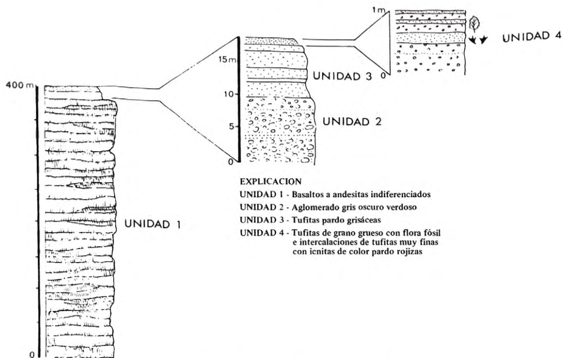
Figura 4. Secuencia estratigráfica de cerro Fósil. (Covacevich y Lamperein, 1970).
