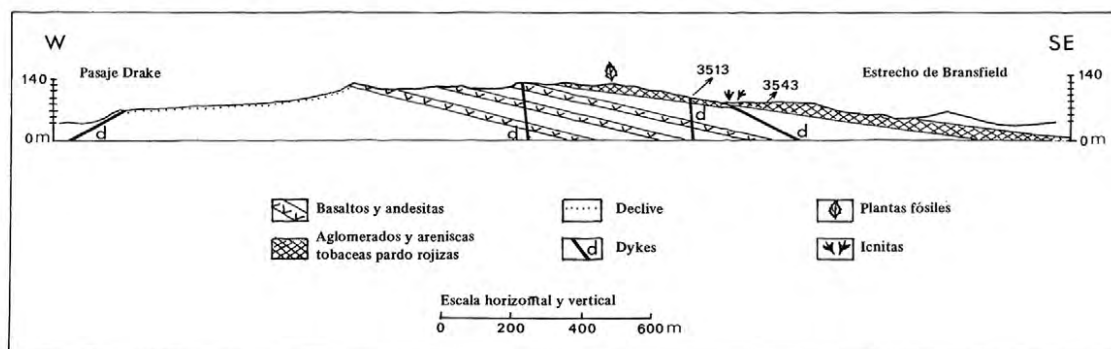
Figura 3. Perfil geológico del cerro Fósil, que indica la unidad de donde provienen los sedimentos portadores de los palinomorfos (tomado de Covacevich y Lamperein, 1970).
