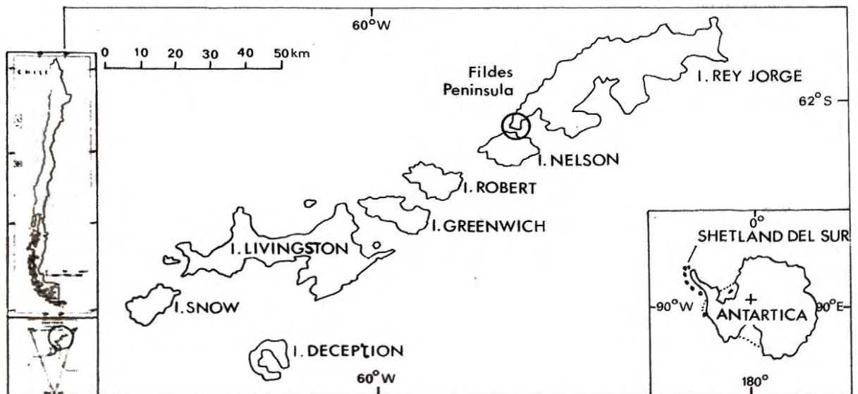
Figura 1. Mapa de ubicación de la isla Rey Jorge. en las islas Shetland del Sur. El círculo muestra la península Fildes, lugar de recolección de las muestras.
