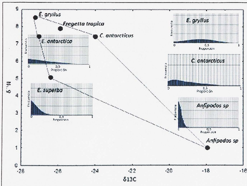
Figura 6. Nicho trófico de F. tropica . Solución obtenida en base a datos conseguidos en el verano de Diciembre del 2009 y Febrero del 2010 y a revisión bibliográfica. Análisis basados en la metodología de Phillips & Gregg 2003. Se incluyen los histogramas de probabilidad de proporción en la dieta para cada presa.
