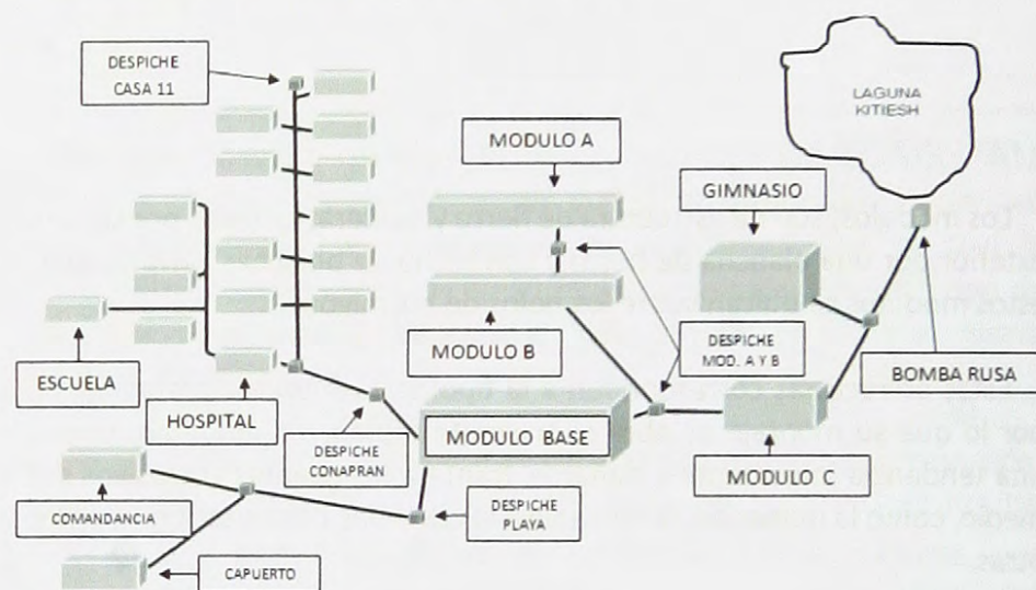
Diagrama de distribución de agua en Base Frei.
