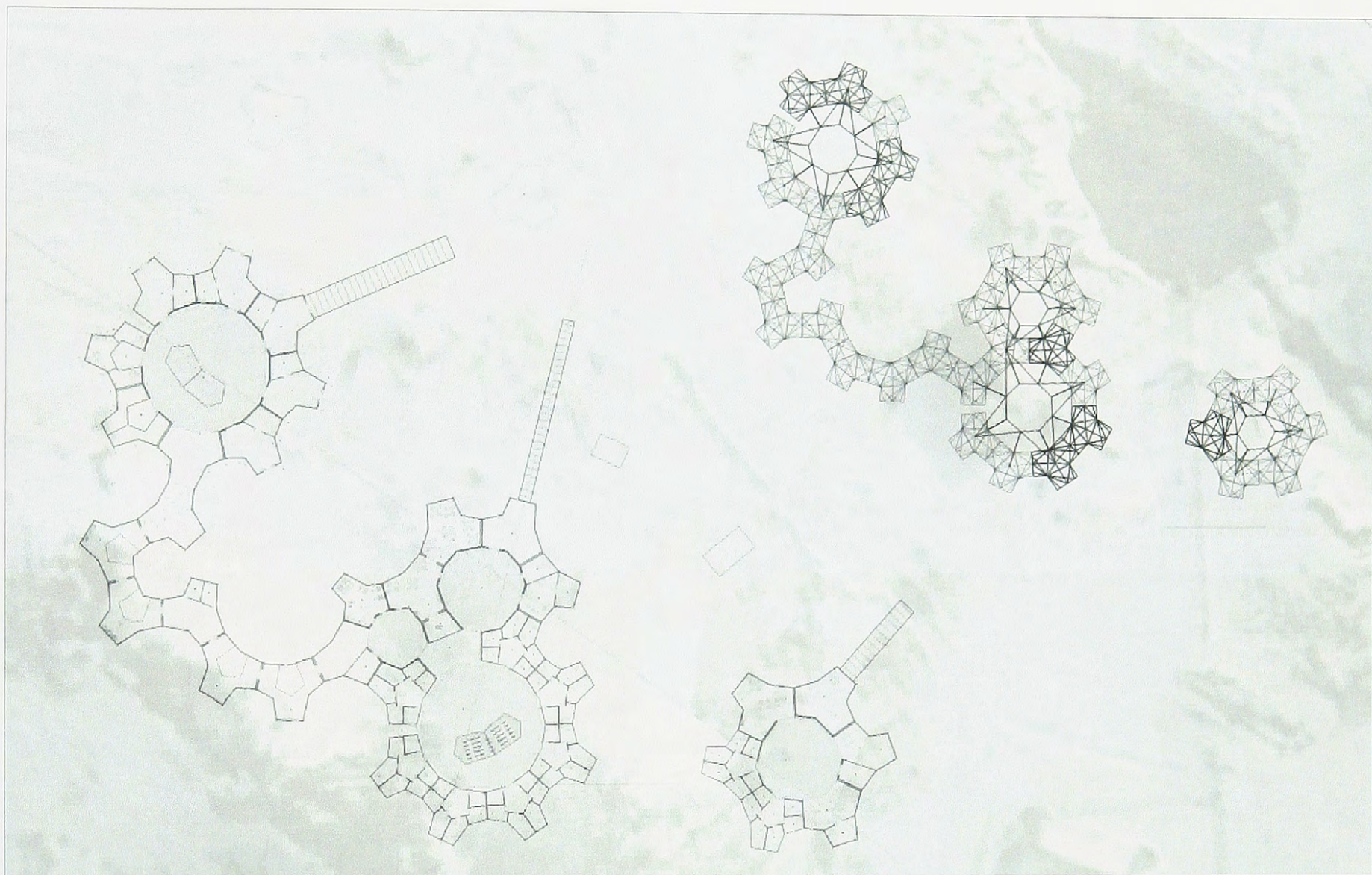
PLANIMETRÍA DE PLANTA Y ESTRUCTURA PROPUESTA DE ESTUDIO DE MÓDULO 1 Fuente: Elaboración propia
