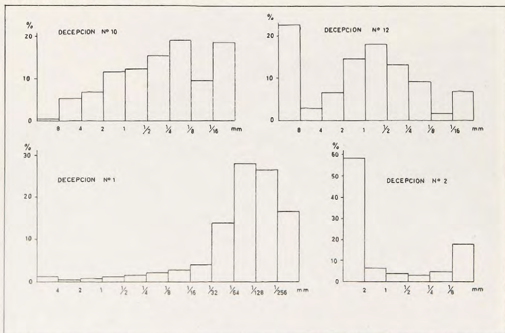
Fig. 3.—Histogramas de frecuencias de muestras de Piroclásticos.
