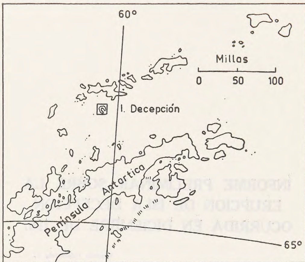
Fig. 1.- Mapa de ubicación de la I. Decepción.
